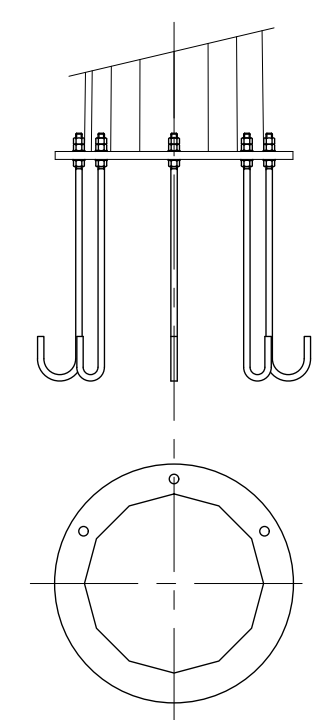
DETALLE PLACA DE BASE
