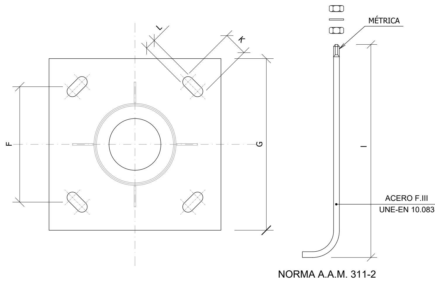
PLACA DE BASE
