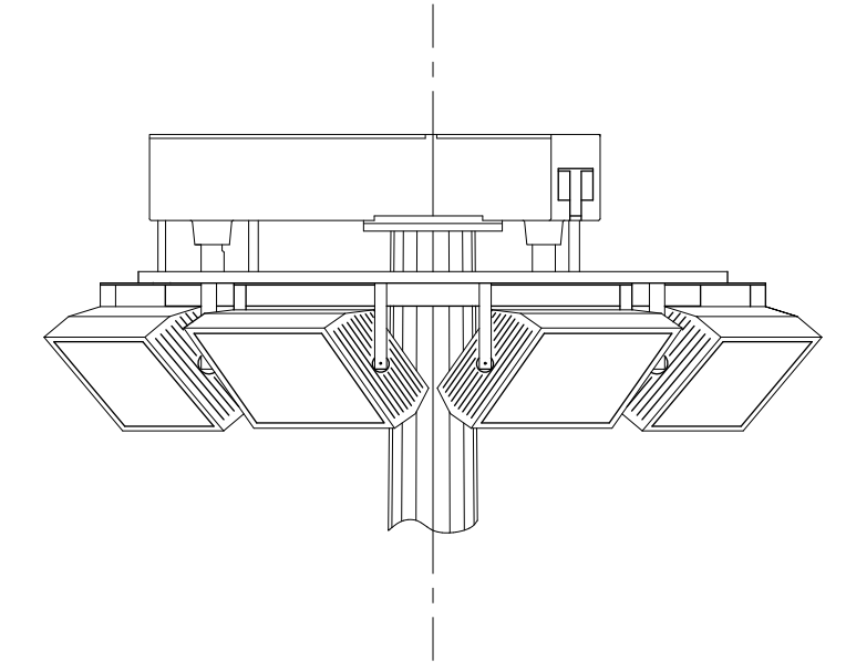
PARTE SUPERIOR DE LA TORRE HASTA n.6 - 8 PROYECTORES A 360°
