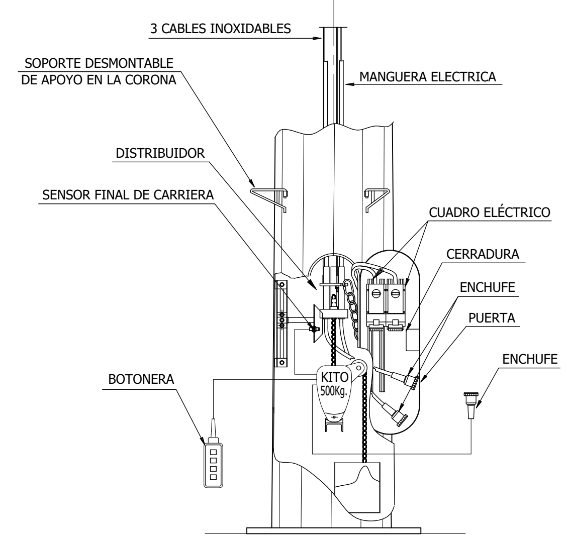
BASE DE LA TORRE MOTOR INTEGRADO
