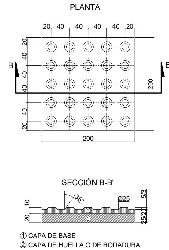
DETALLE BALDOSA TÁCTIL DE BOTONES E: 1/5 Cotas en mm.
