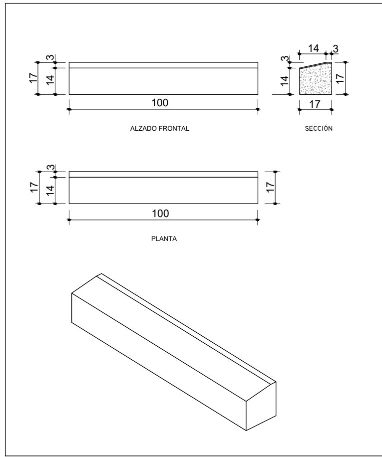
DETALLE BORDILLO BARBACANA CENTRAL E: 1/20 Cotas en cm.
