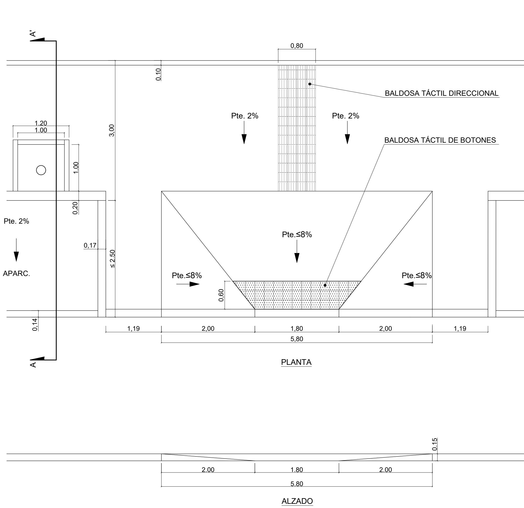
DETALLE BARBACANA PASO DE PEATONES TIPO "A" ESCALA: 1/ 40 Cotas en m.
