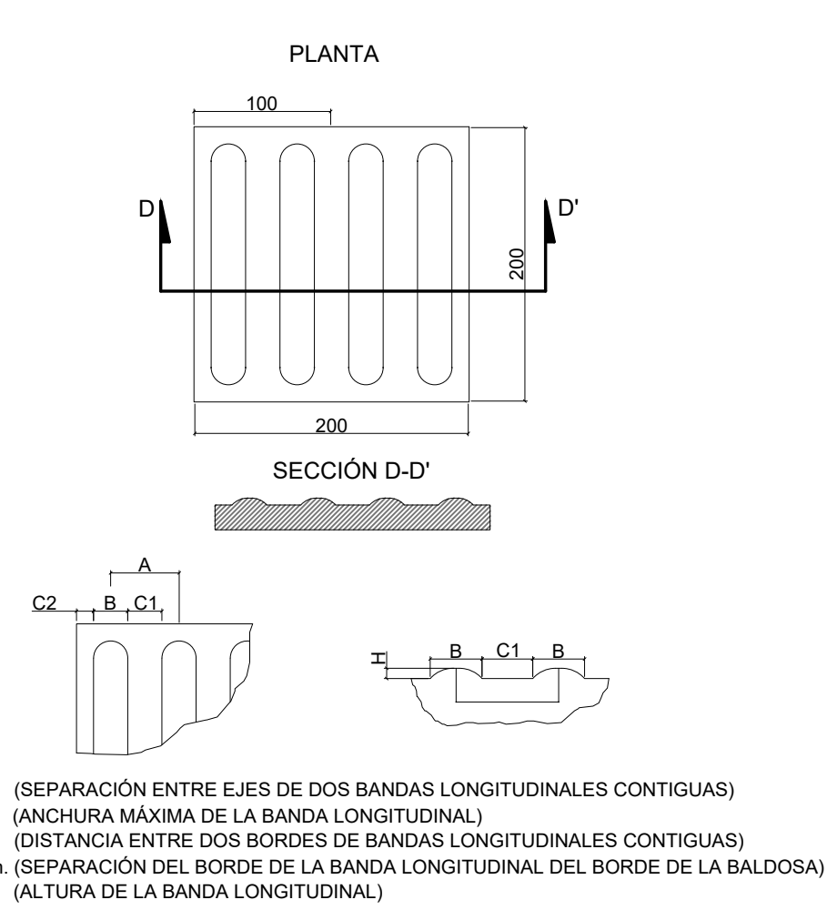
DETALLE BALDOSA TÁCTIL DIRECCIONAL E: 1/5 Cotas en mm.
