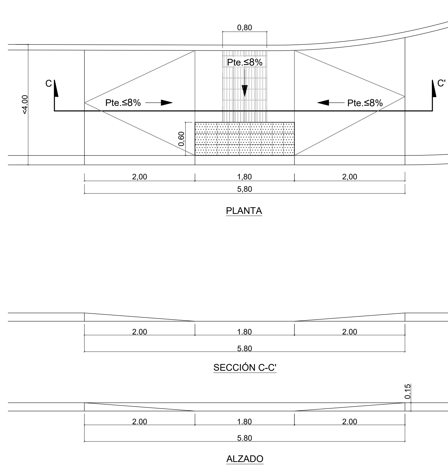
DETALLE BARBACANA PASO DE PEATONES TIPO "B" ESCALA: 1/ 40 Cotas en m.
