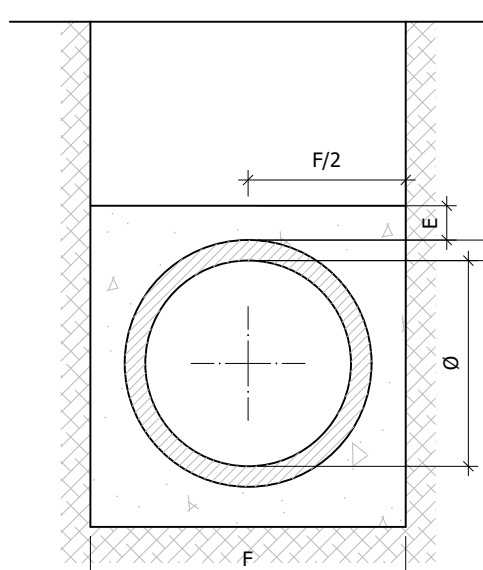
SECCION B-B
