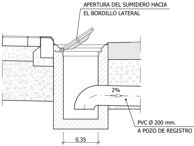
SECCIÓN B-B
