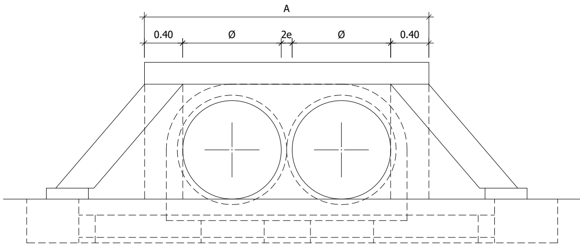
ALZADO
