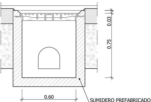
SECCIÓN A-A
