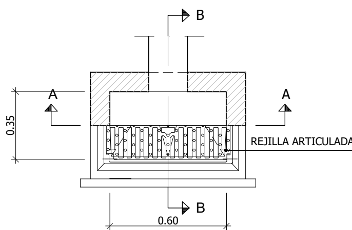
PLANTA SEMI-SECCIÓN
