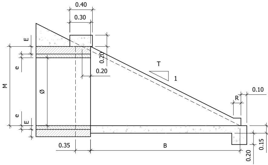
SECCION A-A
