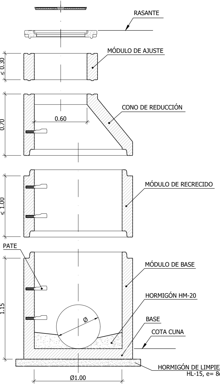
POZO DE REGISTRO Ø1.00 m PREFABRICADO DE HORMIGÓN ARMADO PARA TUBERÍA <Ø0.50 m
