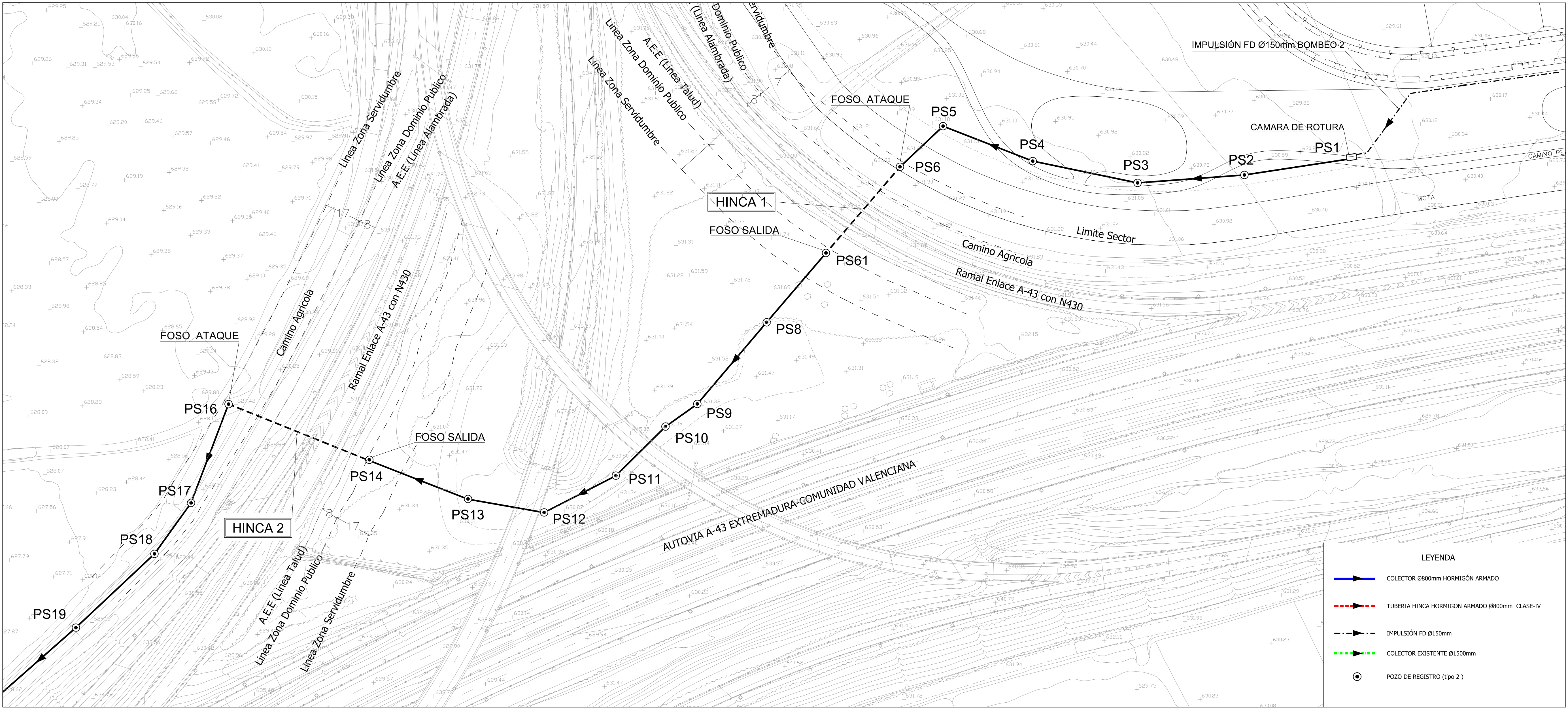
PLANTA COLECTOR CONEXION DE FCALES (PS1-PS19) EH 1/1000
