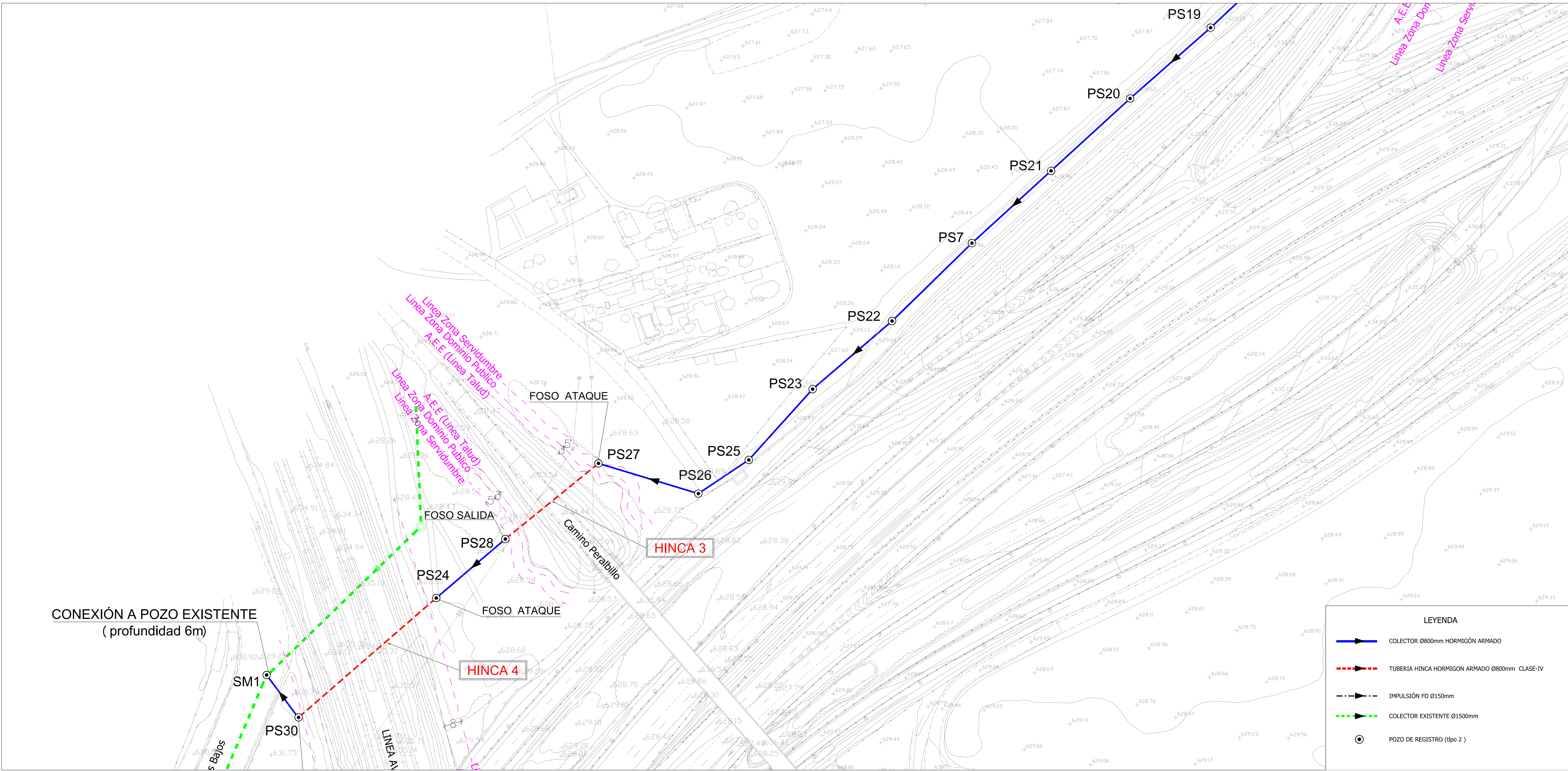
PLANTA COLECTOR CONEXION DE FECALES (PS19-SM1) E1/1000
