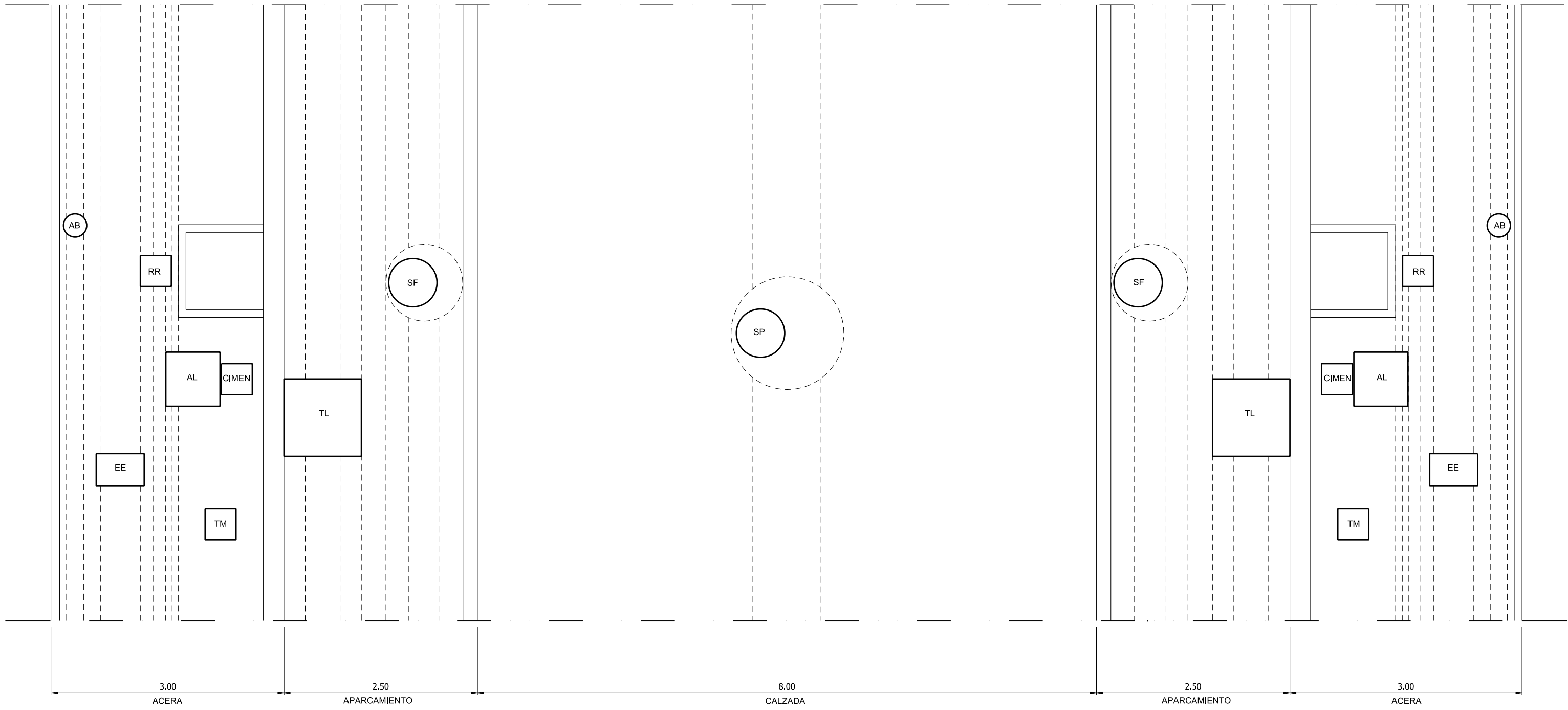
PLANTA DE COMPATIBILIDAD DE ARQUETAS
