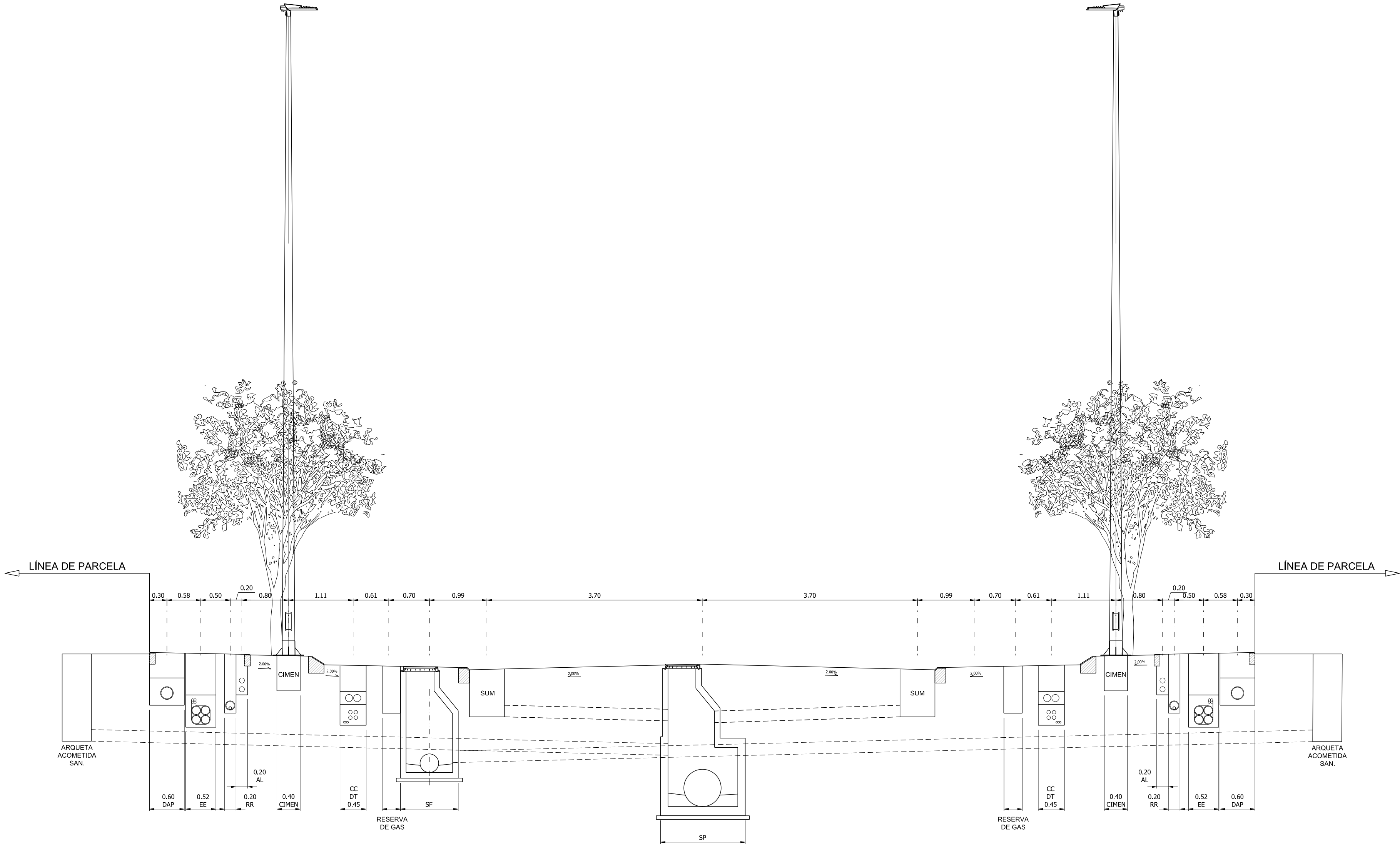
SECCIÓN DE COORDINACIÓN DE SERVICIOS VIAL A
