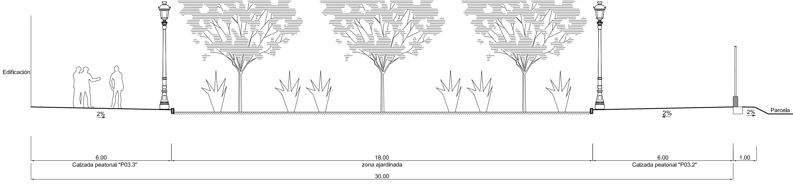
SECCIÓN 11-11 Calles Peatonales "P03.2-P03.3"
