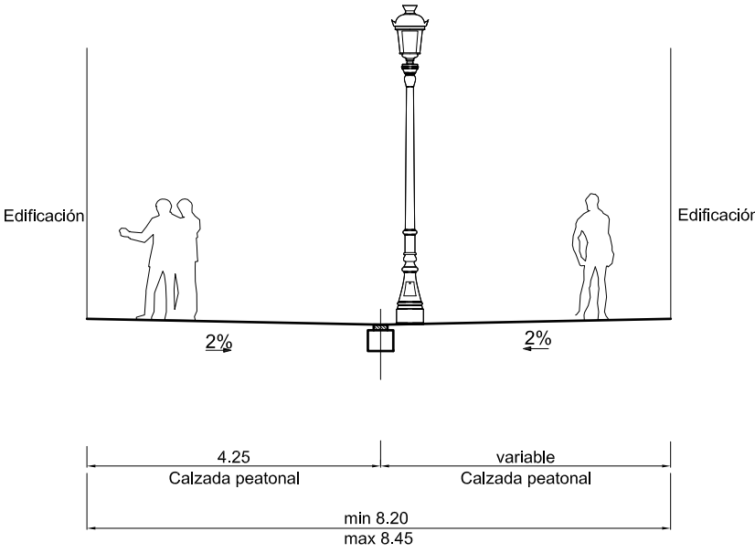
SECCIÓN 10-10 Calle Peatonal "P03.1"
