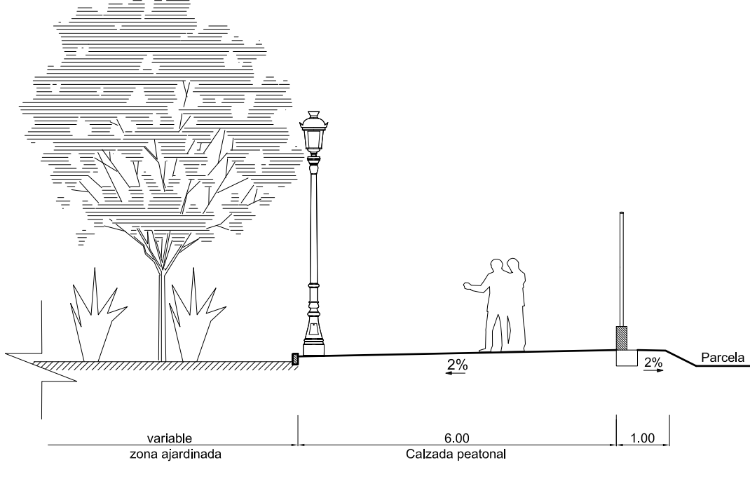
SECCIÓN 13-13 Calle Peatonal "P02"
