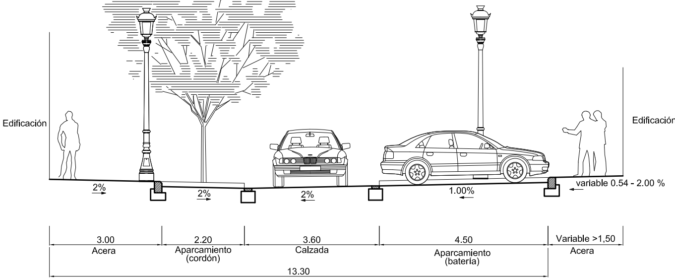
SECCIÓN 7-7 Calle "URUGUAY"
