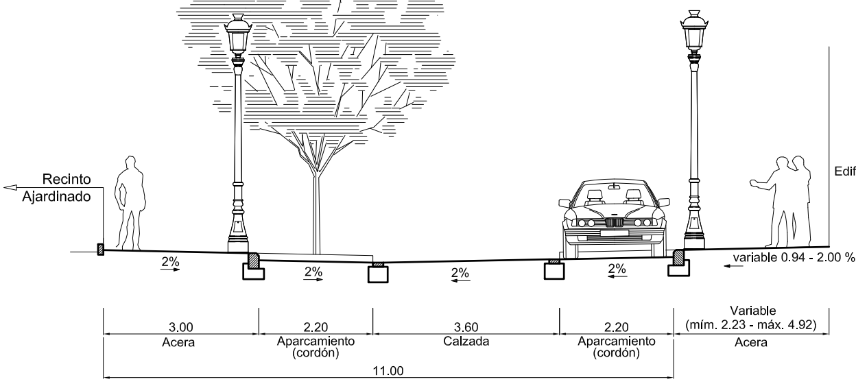
SECCIÓN 8-8 Calle "URUGUAY"
