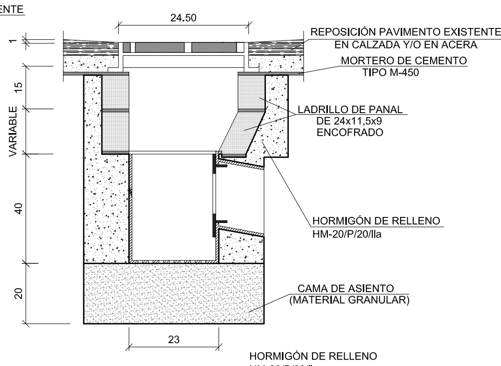
SECCIÓN B-B'
