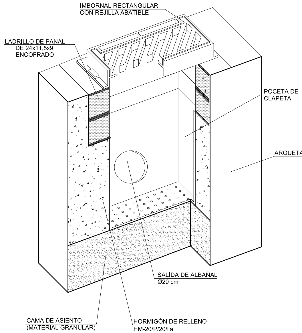
PERSPECTIVA
