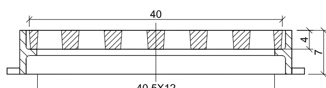
SECCIÓN E-E'
