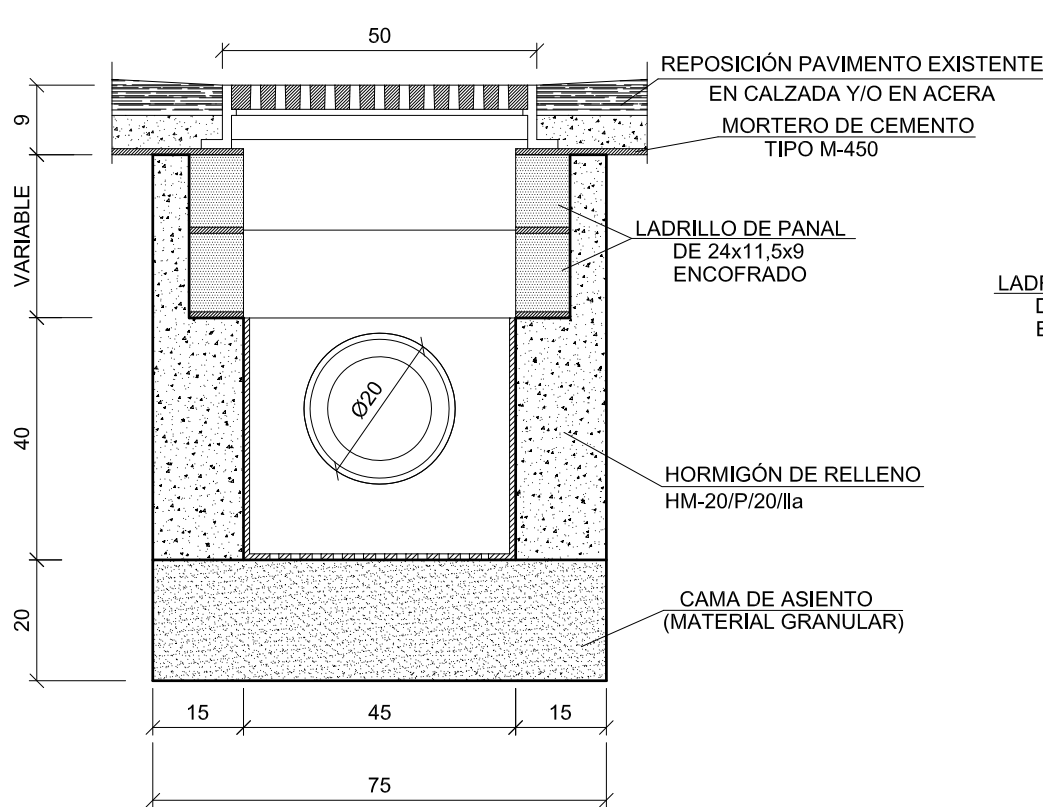
SECCIÓN C-C'
