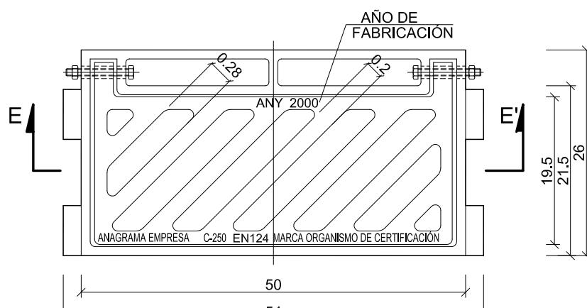
PLANTA
