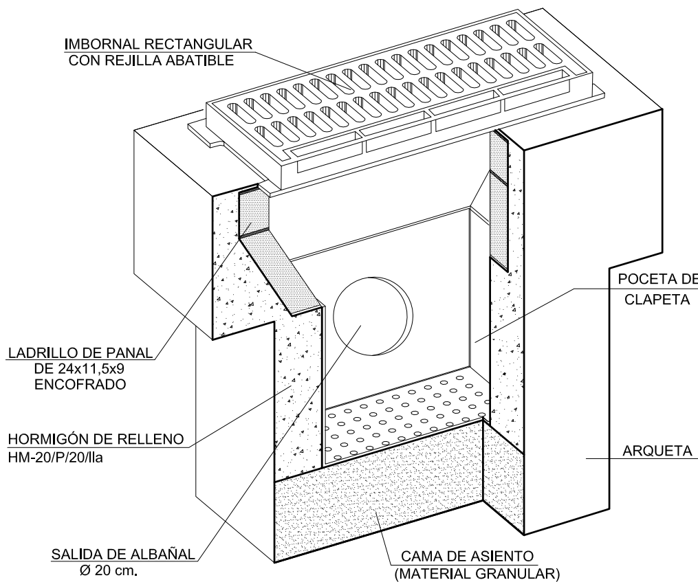
PERSPECTIVA
