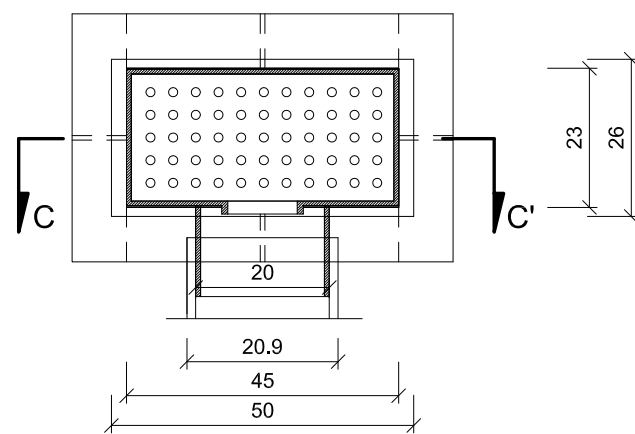
PLANTA
