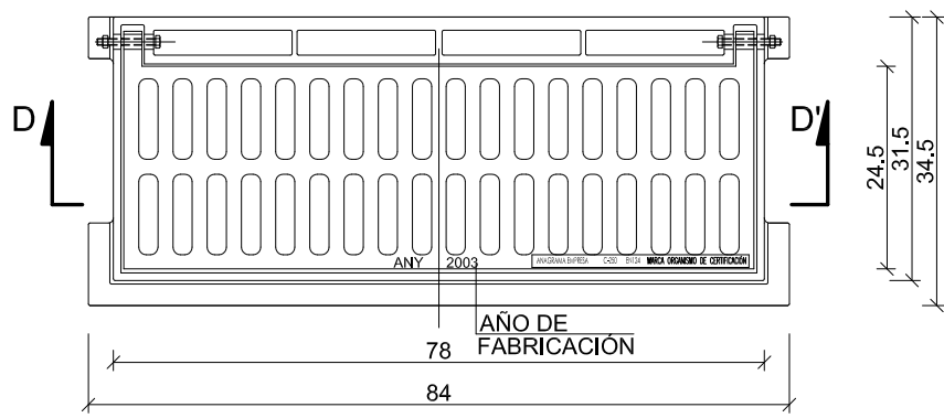
PLANTA
