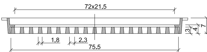
SECCIÓN D-D'
