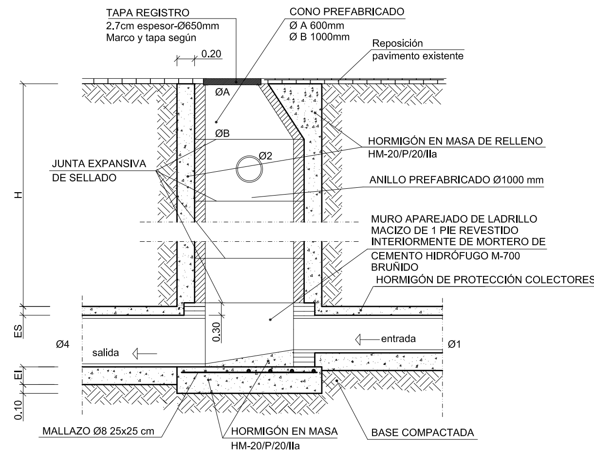
SECCIÓN A-A'
