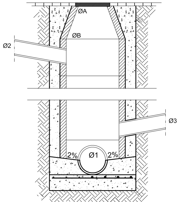
SECCIÓN D-D'
