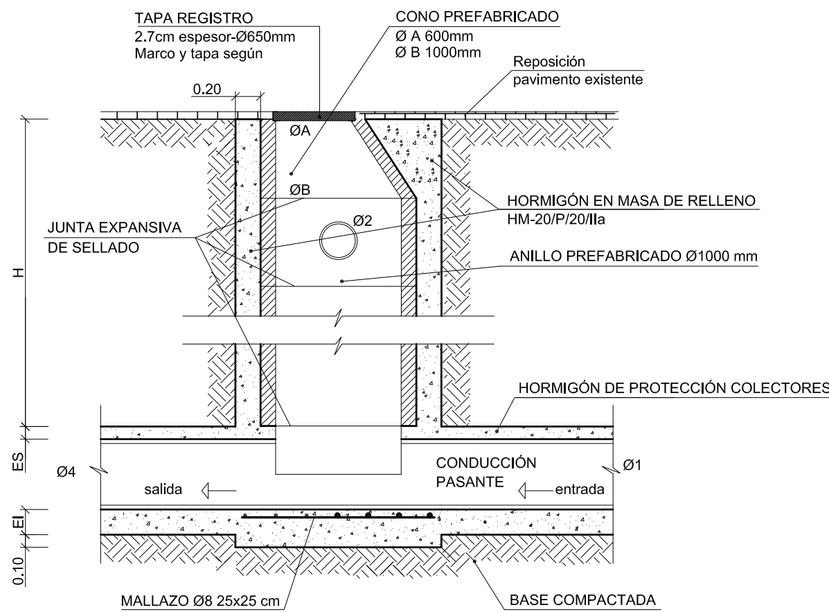
SECCIÓN C-C'
